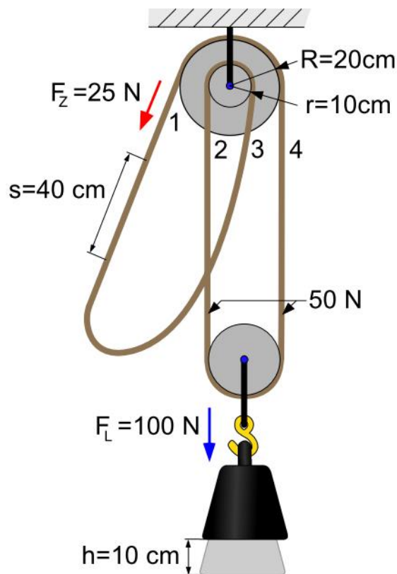
Abb. 11: Differenzialflaschenzug (Quelle: Wikipedia [1])
